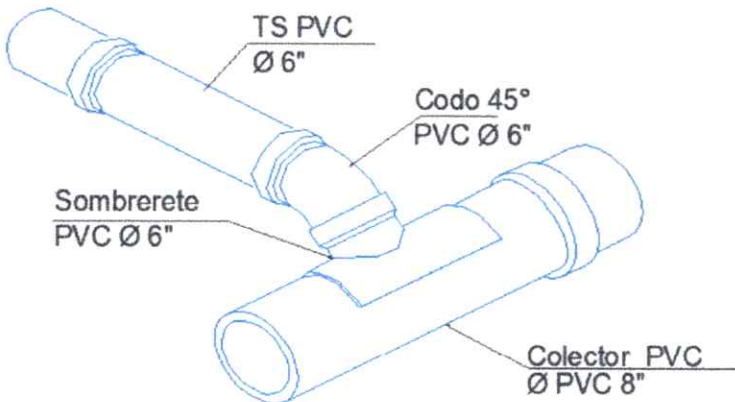
DETALLE CONEXIÓN DOMICILIARIA PERSPECTIVA DE EMPALME A LA RED
