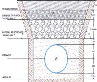
DETALLE DE CIMENTACION PARA VIAS PAVIMENTADAS TIPO C3
