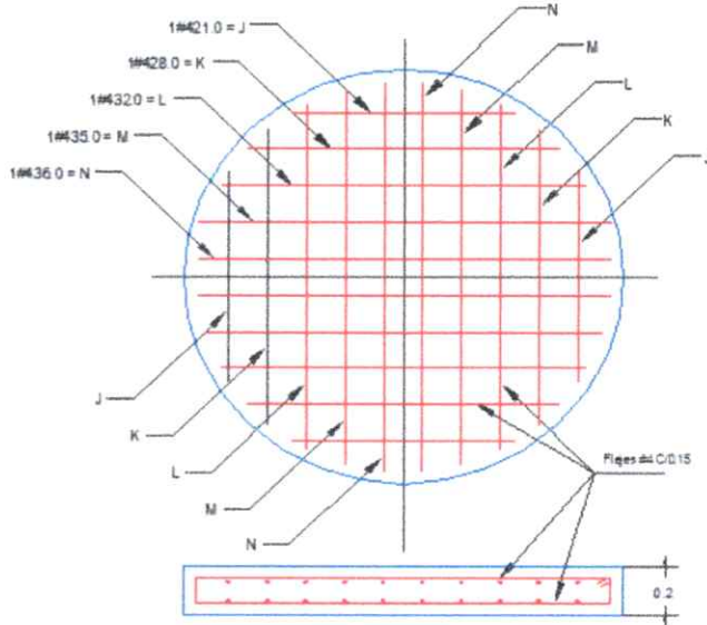
REFUERZO PLACA BASE
