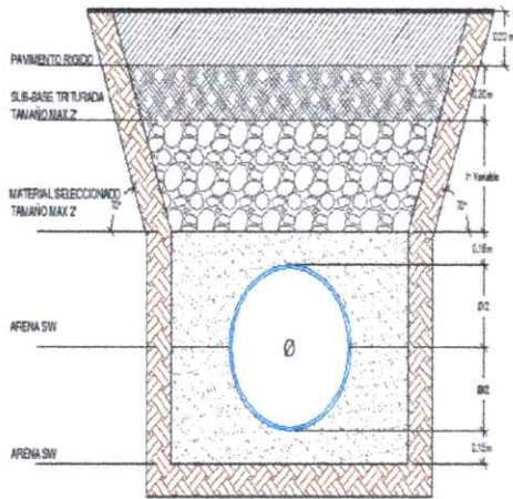
DETALLE DE CIMENTACION PARA VAS PAVIMENTADAS TIPO C3
