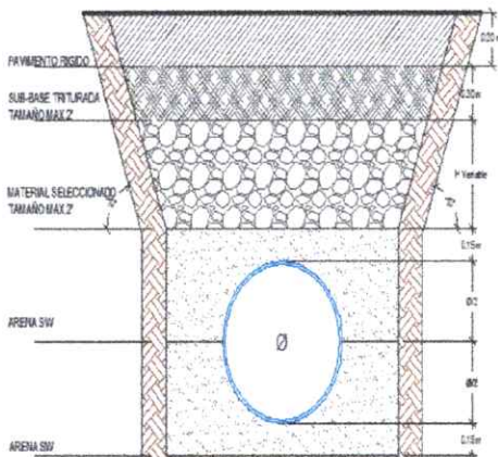
DETALLE DE CIMENTACION PARA VIAS PAVIMENTADAS TIPO C3
