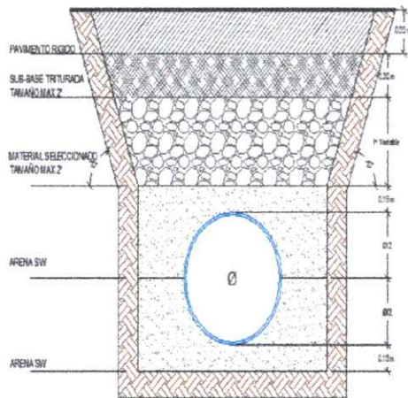
DETALLE DE CIMENTACION PARA MAS PAVIMENTADAS TIPO C3
