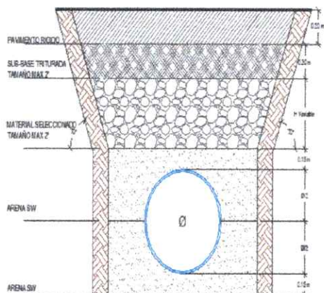
DETALLE DE CIMENTACION PARA MAS PAVIMENTADAS TIPO C3
