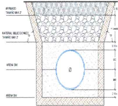
DETALLE DE CIMENTACION PARA VIAS SIN PAVIMENTAR TIPO C1
