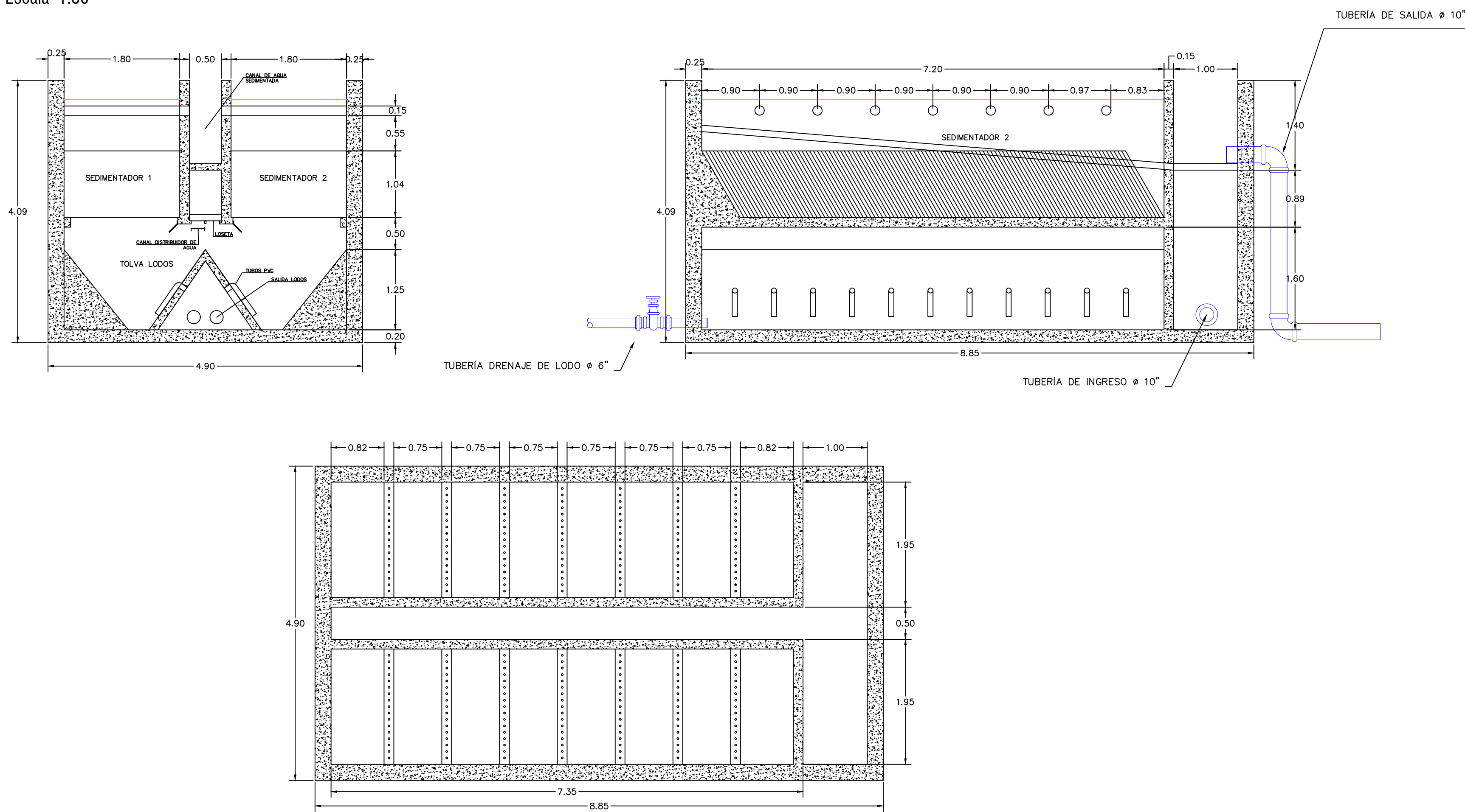
Detalle Sediementador Escala 1:50
