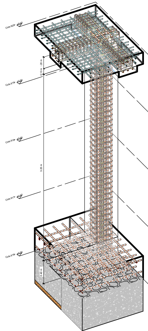
8 DETALLE ISOMETRICO COLUMNA
