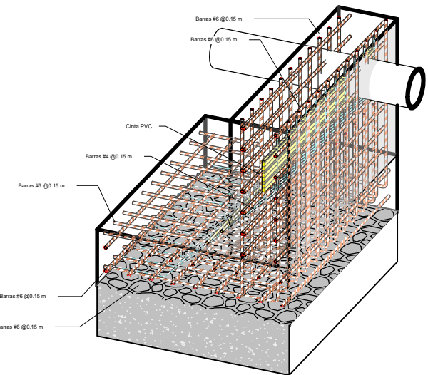
6 DETALLE ISOMETRICO DE REFUERZO NODO INFERIOR
