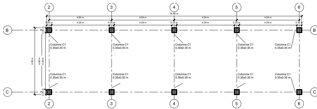
1 PLANTA DE COLUMNAS 1 : 50
