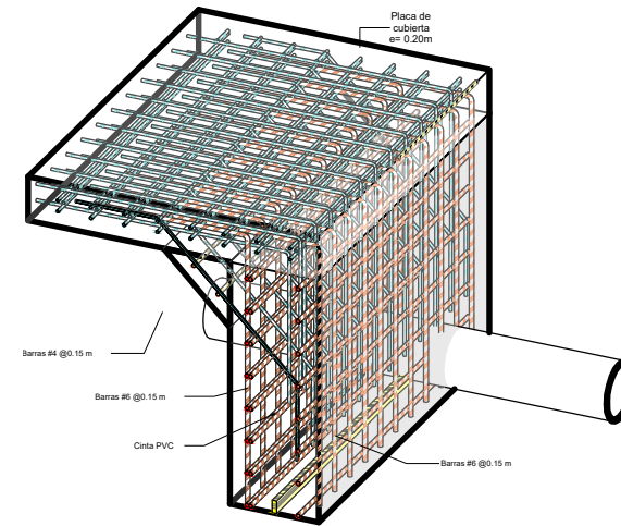
7 DETALLE ISOMETRICO DE REFUERZO NODO SUPERIOR
