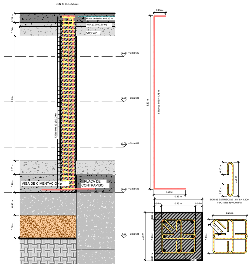
2 DESPIECE DE COLUMNA C1 1 : 15
