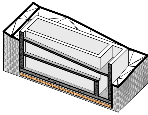
5 Corte Isometrico Longitudinal
