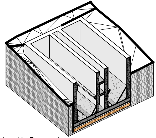
6 Corte Isometrico Transversal
