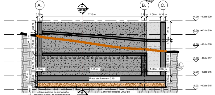
3 Seccion Longitudinal Sedimentador 1: 50
