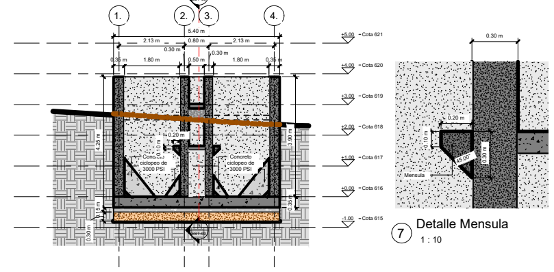
4 Seccion transversal Sedimentador 1: 50
