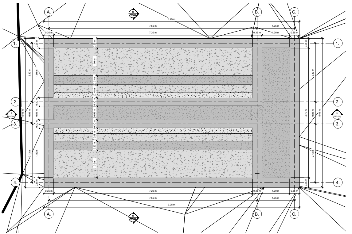
2 Emplazamiento Sedimentador 1: 25
