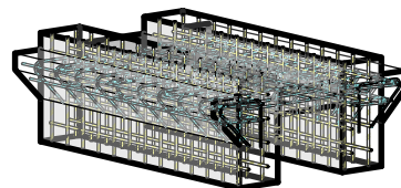
40 Isometrico detalle (mensulas)
