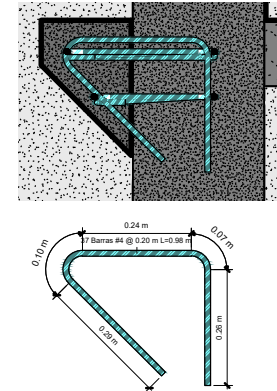
10 Detalle refuerzo Mensula 1:5
