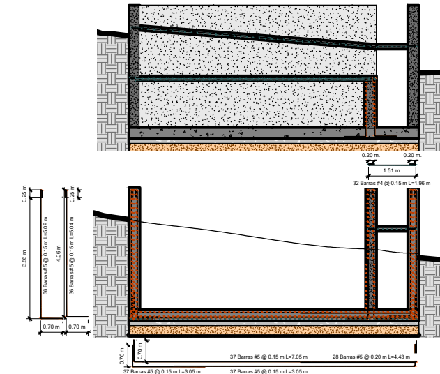
1 Seccion Longitudinal Detalle de Acero 1:50
