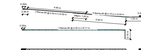
7 Seccion transversal Sedimentador Detalle de Acero 1:50
