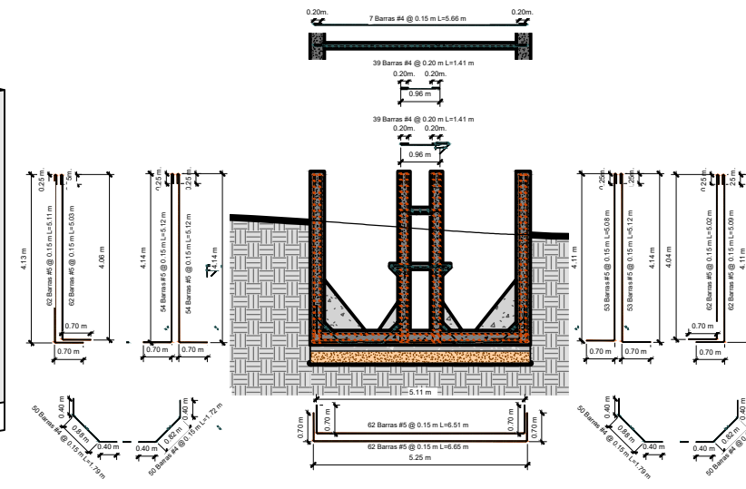
7 Seccion transversal Sedimentador Detalle de Acero 1:50
