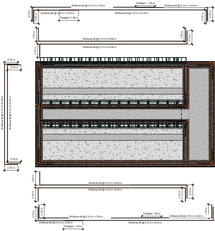
13 DESPIECE ACERO PLACA DE PISO SEDIMENTADOR 1:35
