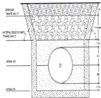
DETALLE DE CIMENTACION PARA MAS SIN PAVIMENTAR TIPO C1
